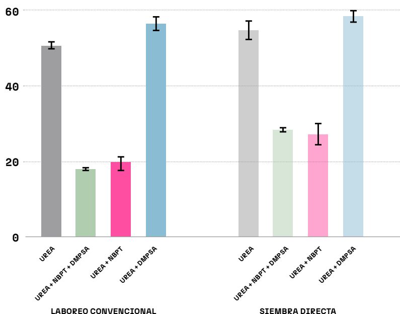
PÉRDIDAS POR VOLATILIZACIÓN DE AMONIACO (kg NH_3 -N/ha)
